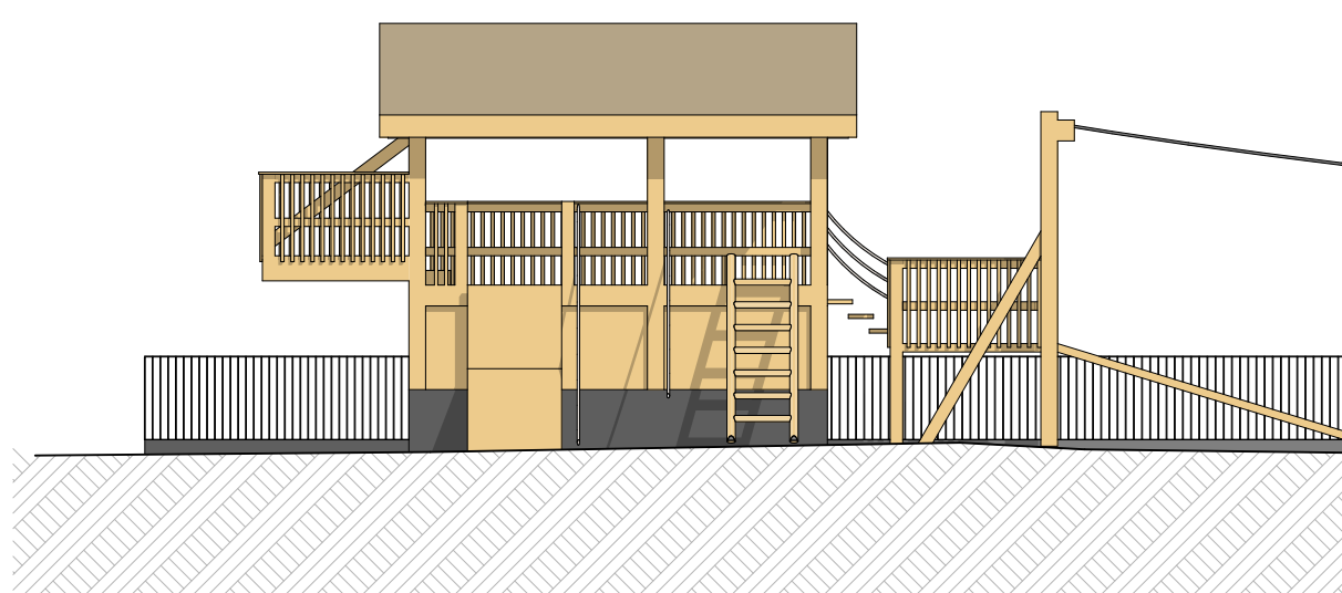
containerhaus ansicht nord
