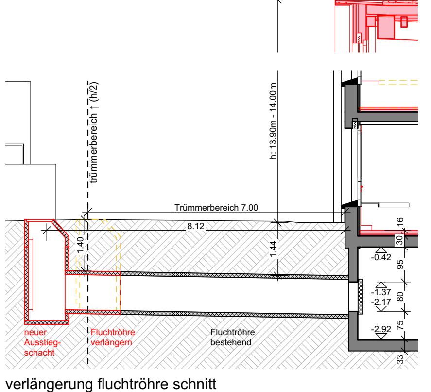
verlängerung fluchtröhre schnitt
