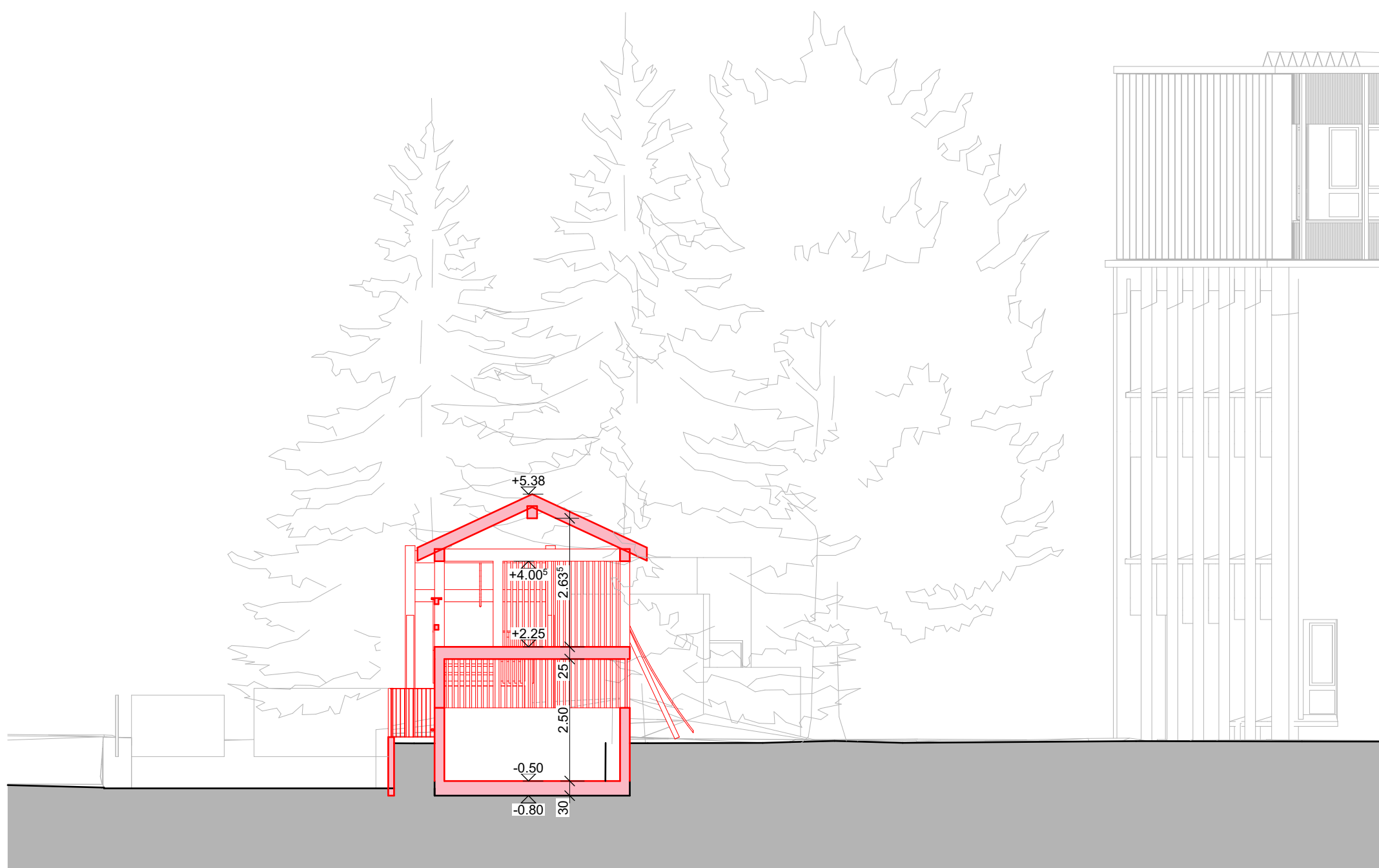
containerhaus querschnitt
